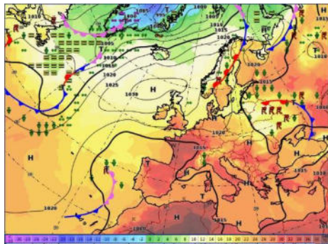
Hochdruckrandlage zweite Julidekade, BWK 11. Juli, DWD
