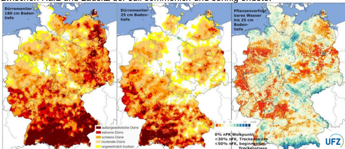
Bodenfeuchte in verschiedenen Bodentiefen am 20. Juli 2026. Bilder: Dürremonitor des UFZ
