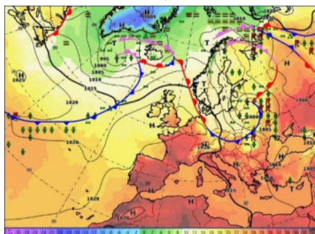
Trogwetterlage während der ersten Julidekade, BWK 08. Juli, DWD
