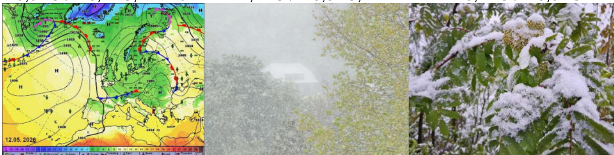
Eine Troglage brachte mit polaren Luftmassen um die Eisheiligen (10. bis 17. Mai) nochmals nassen Schnee und wiederholte nächtliche Luftfröste
