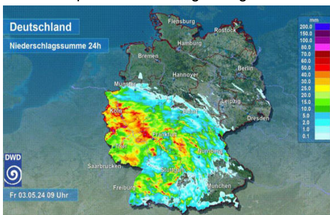
Niederschlagssummen 02./03. Mai 2024
